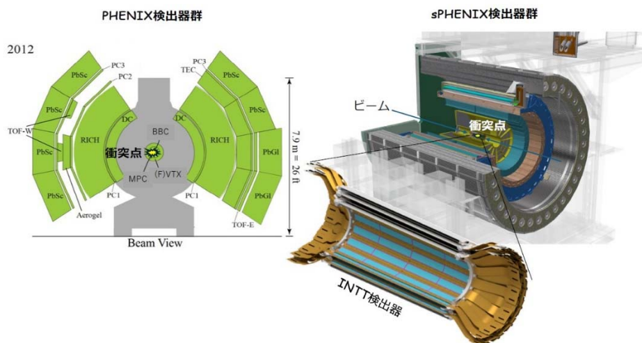
図1 PHENIX 検出器群と sPHENIX 検出器群
